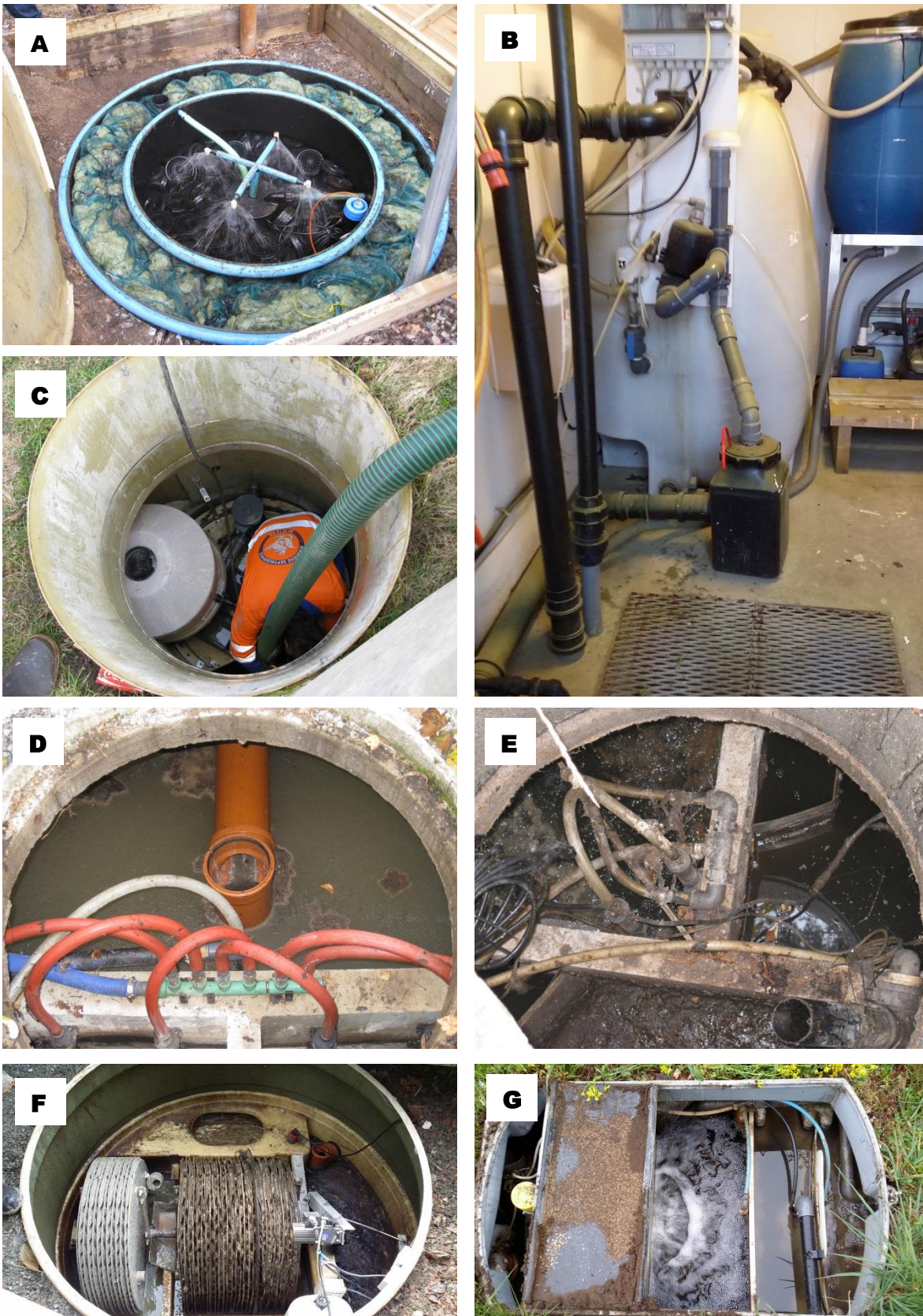
Figur 8: Minirensanlegg kan ha mange ulike utforminger. A) Green Rock minirensanlegg med dyser innerst og steinull i ytre ring. B) Innomhus Biovac-anlegg. C) Rengjøring av Wallax-anlegg. D) Ipec-anlegg. E) Klaro-anlegg. F) Klargester-anlegg med biorotorer. G) Ecobio / Weho-anlegg i luftefase. Det finnes enda flere leverandører på markedet, bl.a. August, Baga og Odin.
